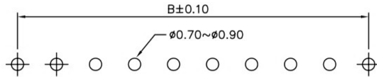
P.C.B. Layout
